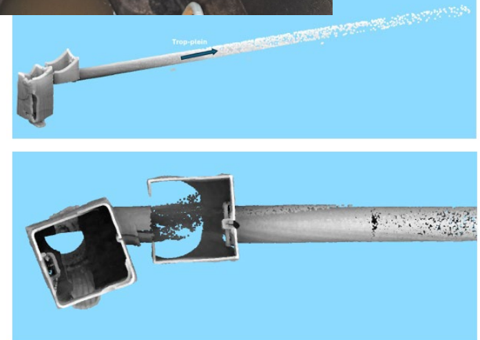
Figure 2-5. Résultats du scan 3D : Vue d'ensemble de l'ouvrage (en haut) et vue de la chambre de déversement (en bas) (Source : 3D EAU).
